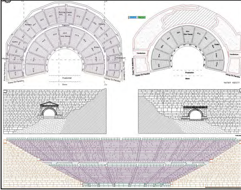
Şekil 5: Tiyatro Restitüsyon
