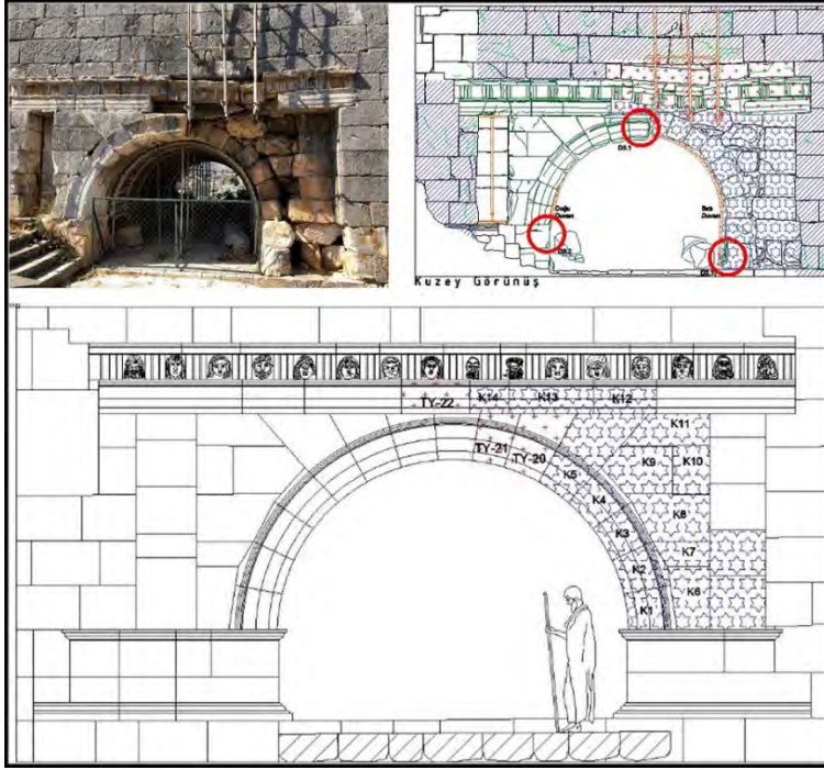
Şekil 6: Tiyatro Restorasyon
