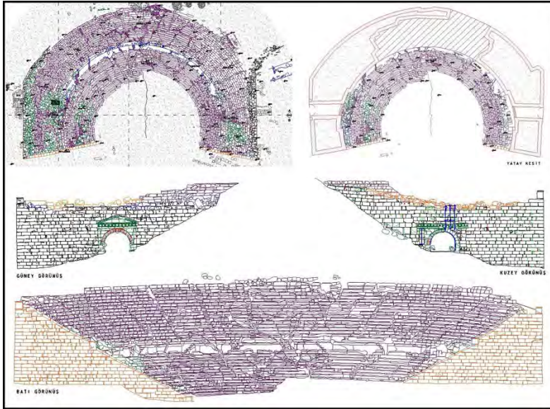
Şekil 4: Tiyatro Rölöve
